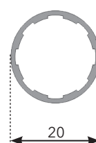
Coupe du tube (de 161 cm à 230 cm de haut)
