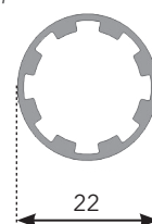
Coupe du tube (jusqu'à 160 cm de haut)
