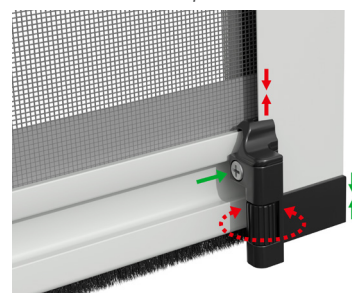
Pied réglable
